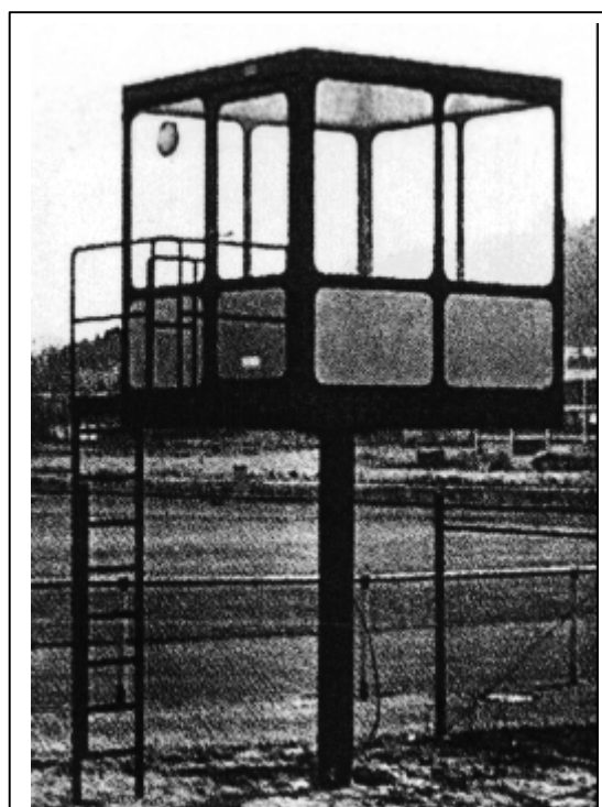
Zielturm ZT 08 / Event Tower ZT 08 Maße/Size: 2,22 x 2,22x 2,60 m Höhe/Height: 5 m
